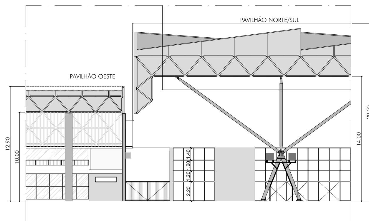
DET. PAVILHÃO OESTE/PAVILHÃO NORTE SUL esc. 1:250
