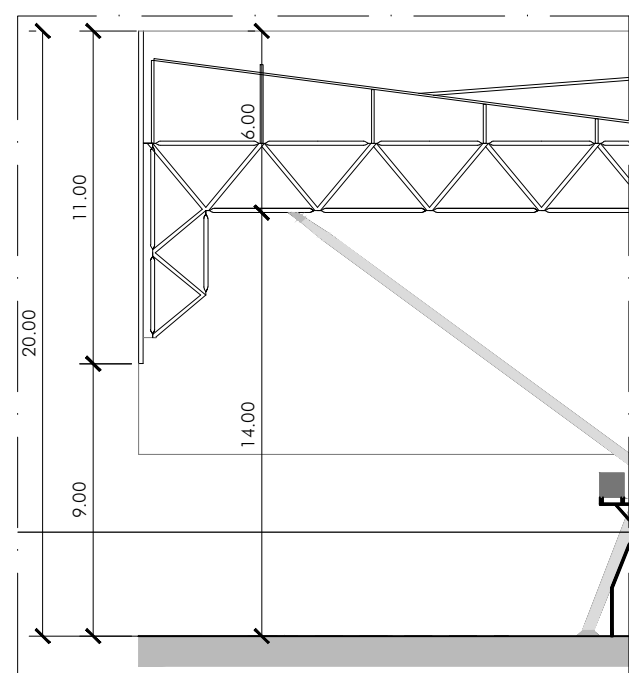
CORTE TÍPICO FACE OESTE DO PAVILHÃO NORTE/SUL esc. 1:250
