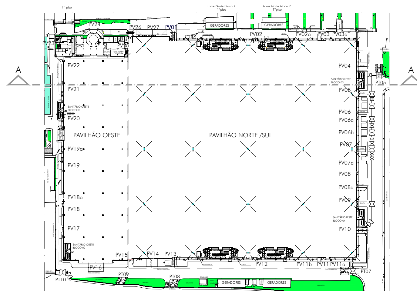
PLANTA esc. 1:2500
