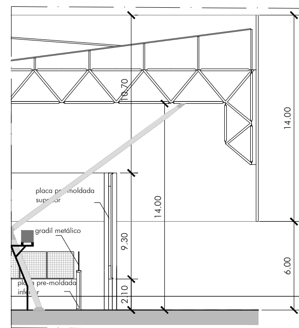
CORTE TÍPICO FACE NORTE, SUL E LESTE DO PAVILHÃO NORTE/SUL esc. 1:250
